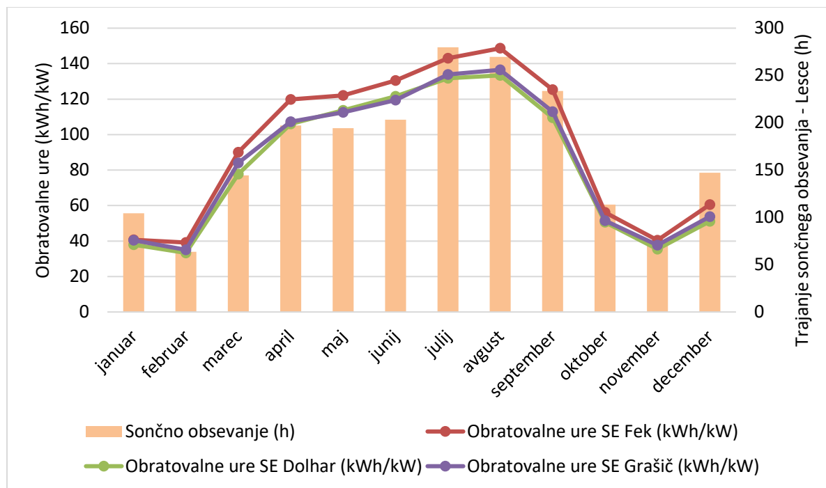
Slika 3: Primerjava trajanja sončnega obsevanja in obratovalnih ur v sončnih elektrarnah Vir: ARSO, lastni izračuni
